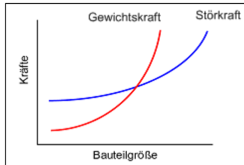
Abbildung 2: Relevante Kräfte in Abhängigkeit von der Bauteilgröße
